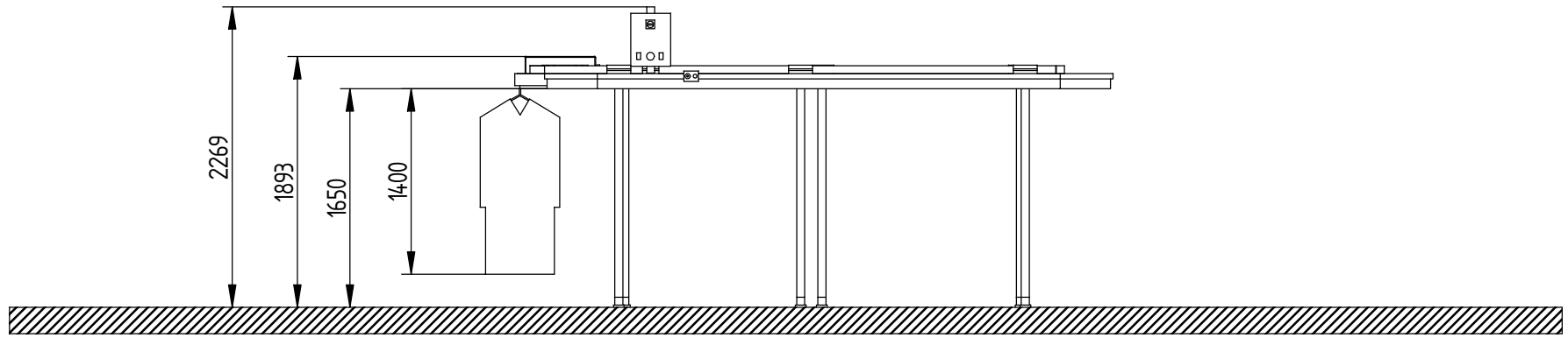
SEZIONE A-A
