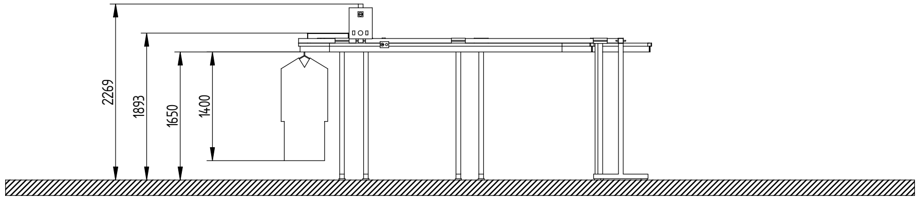
SEZIONE A-A
