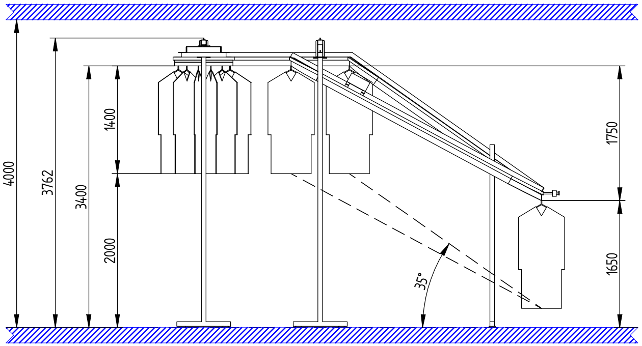
View A-A
