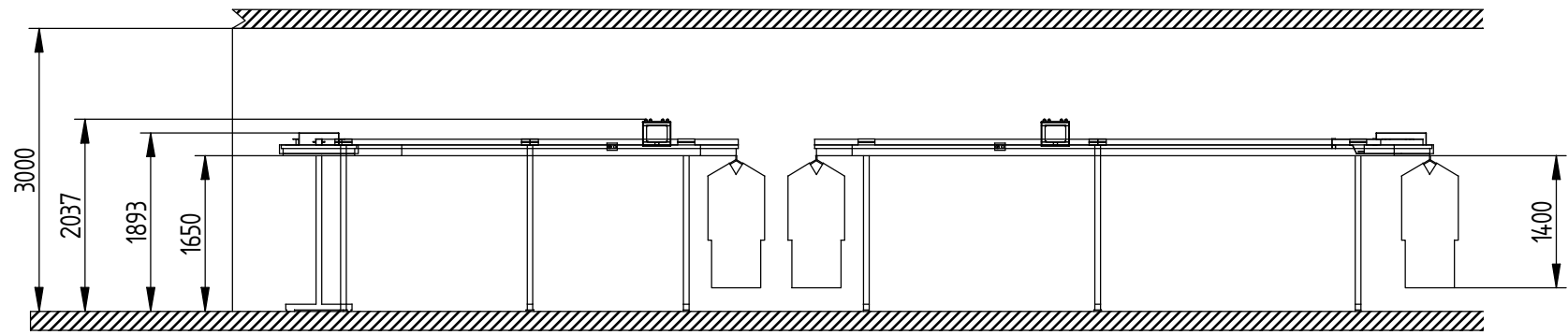
VIEW A-A
